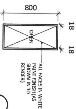
5 FRONT VIEW S-9.2 SCALE: 1:30M
