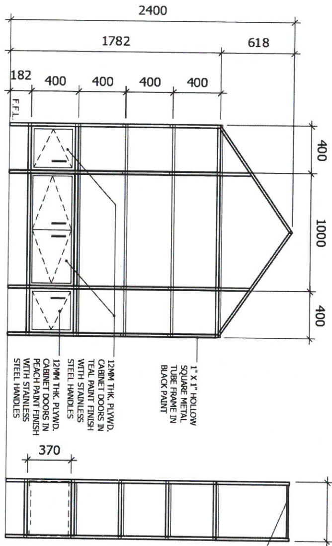
2 FRONT VIEW S-4 SCALE: 1:30M
