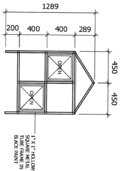
2 FRONT VIEW S-7 SCALE: 1:30M
