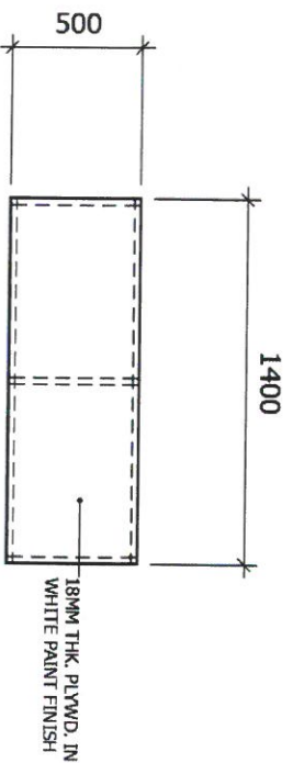
1 TOP VIEW S-3 SCALE: 1:30M
