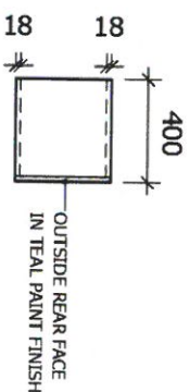
3 RIGHT SIDE VIEW S-9.2 SCALE: 1:30M
