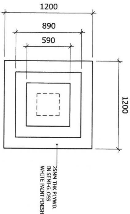
1 TOP VIEW S-11 SCALE: 1:30M
