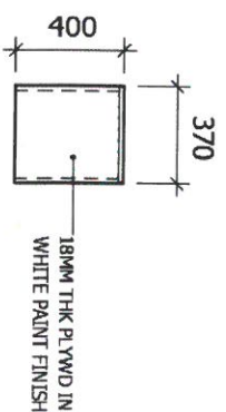
4 TOP VIEW S-9.2 SCALE: 1:30M
